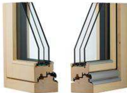
Il nuovo serramento Clima 92 Complanare Certificato Arca "Gold Plus"
